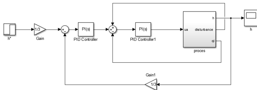
Figura 4.12 Schema bloc a sistemului de reglare în cazădă și cu structură de tip feed-forward
