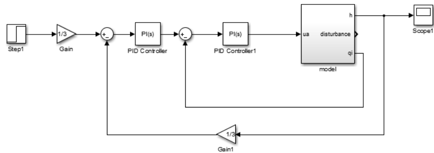
Figura 4.9 Schema bloc pentru reglarea în cascadă
