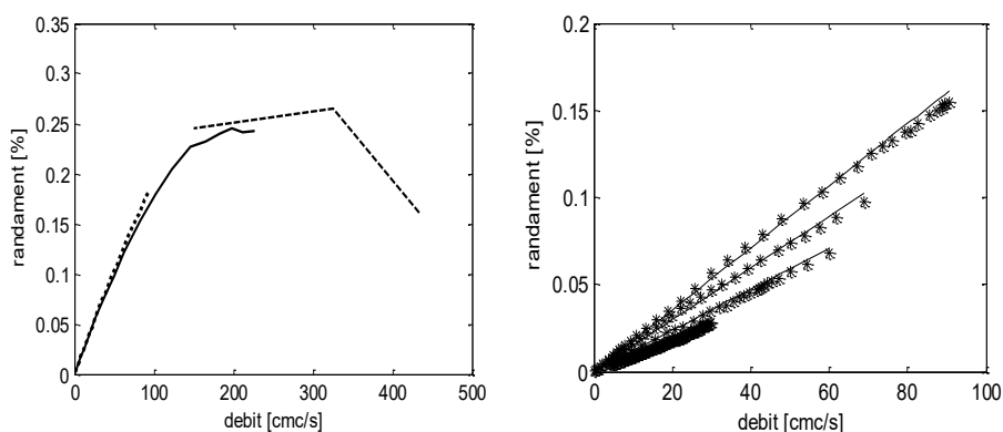
Figura 2.7 Randamentul pompei centrifuge (stânga); Liniarizarea randamentului (dreapta)
