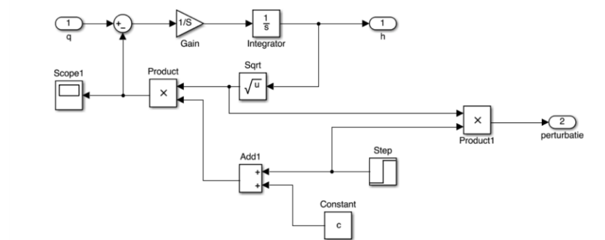
Figura 4.1 Introducerea perturbației pe debitul de ieșire.
