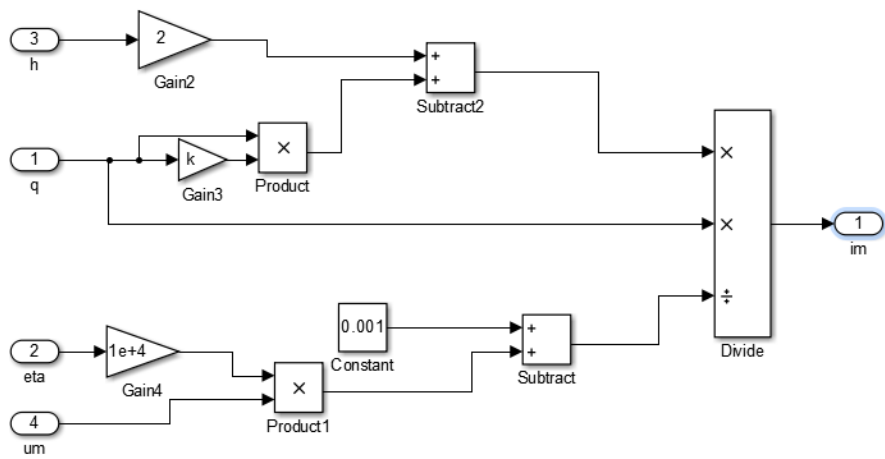
Figura 2.9 Schema Simulink pentru calculul curentului rotoric
