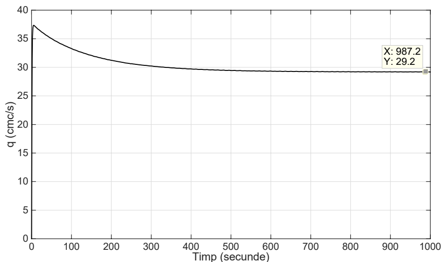
Figura 3.2 Evoluția debitului la o intrare treaptă u_a = 5V
