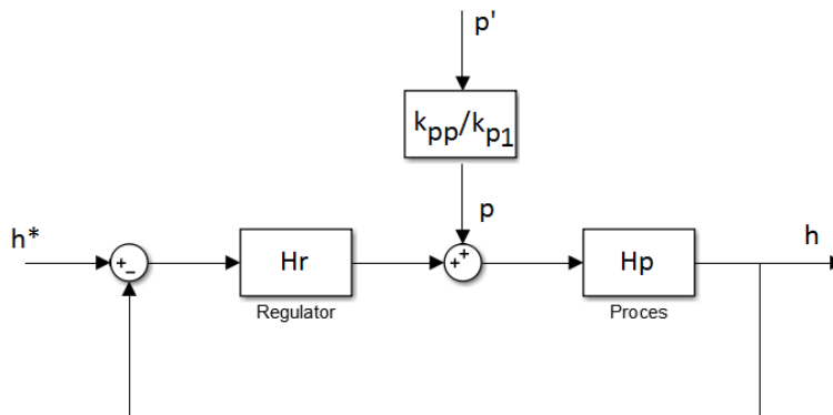
Figura 3.10 Schema de reglare clasică
