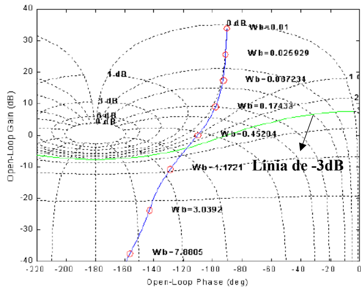
Figura 3.15 Reprezentarea benzii de trecere w_b pe diagrama Nichols
