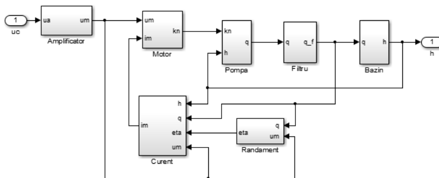
Figura 2.17 Schema bloc a instalației cu filtru
