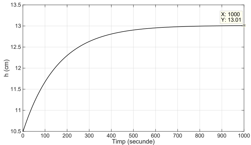
Figura 3.3 Ieșirea sistemului ( h ) la o modificare a intrării de 0.5\text{ V}
